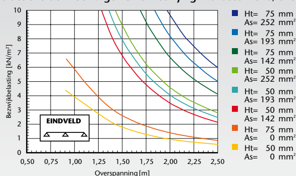
Grafiek 60 minuten brandwerendheid van de LEWIS® constructieve dekvloer afgewerkt met fijn grind beton C20/C25.
